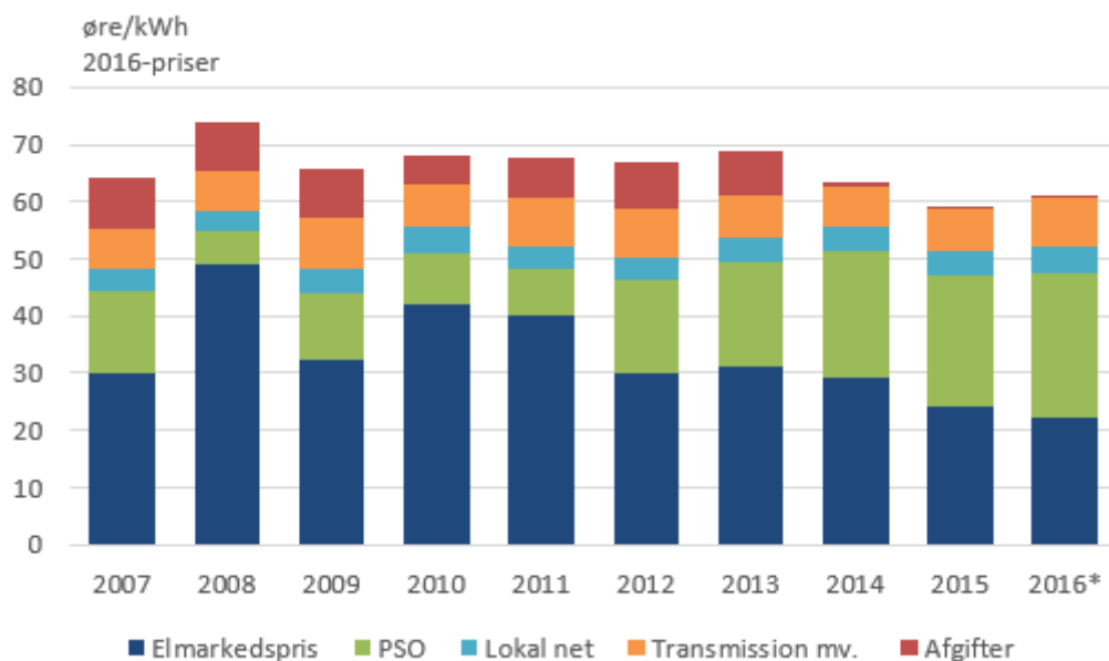
Figur 3. Elprisen for erhverv i forbrugsinterval 20-70 GWh
